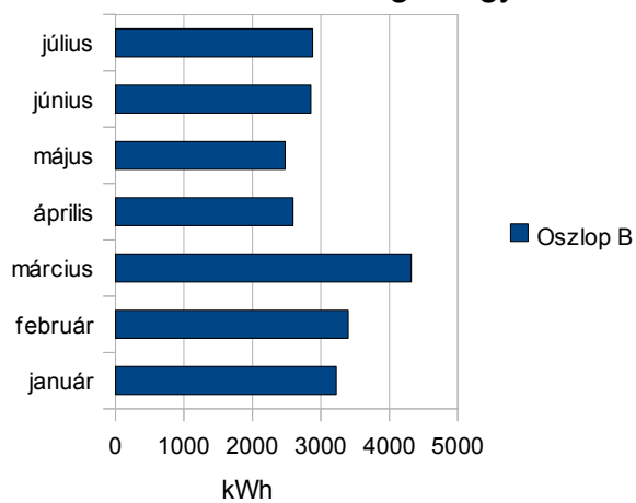
2010 évi villamos energia fogyasztás
